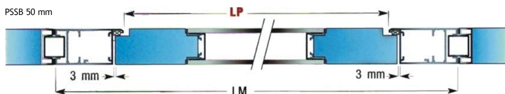
Przekrój przez skrzydło drzwiowe z przeszkleniem i ościeżnicę
