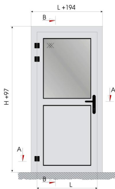
Współpłaszczyznowość ościeżnicy i skrzydła drzwi
