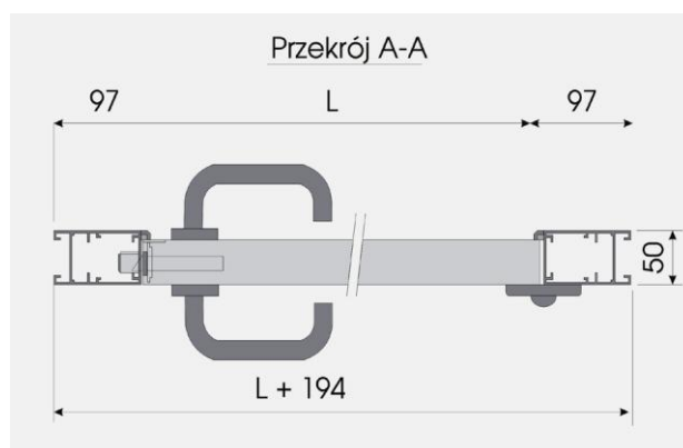
Detal połączeń okna, maskownicy i skrzydła drzwi
